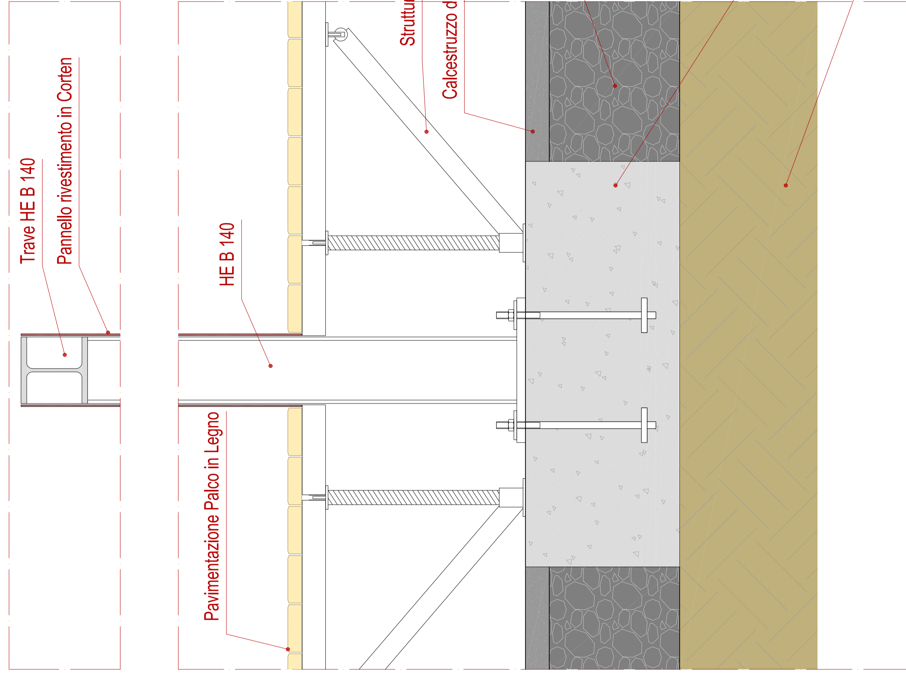
DETTAGLIO A - scala 1:5
